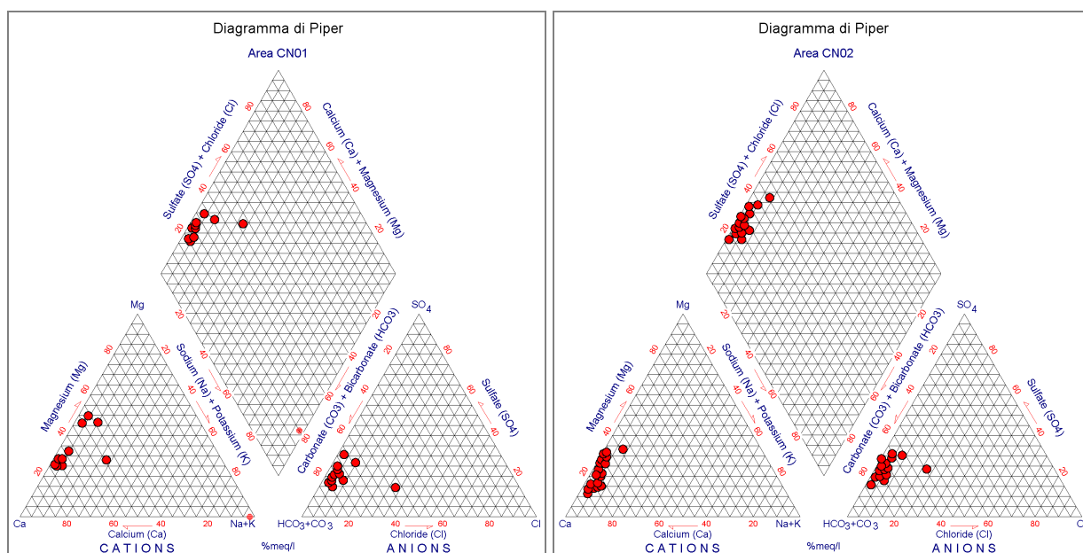
Figura 4.38: Diagramma di Piper delle Aree Idrogeologiche CN01 e CN02 assimilabili al GWB-S6
