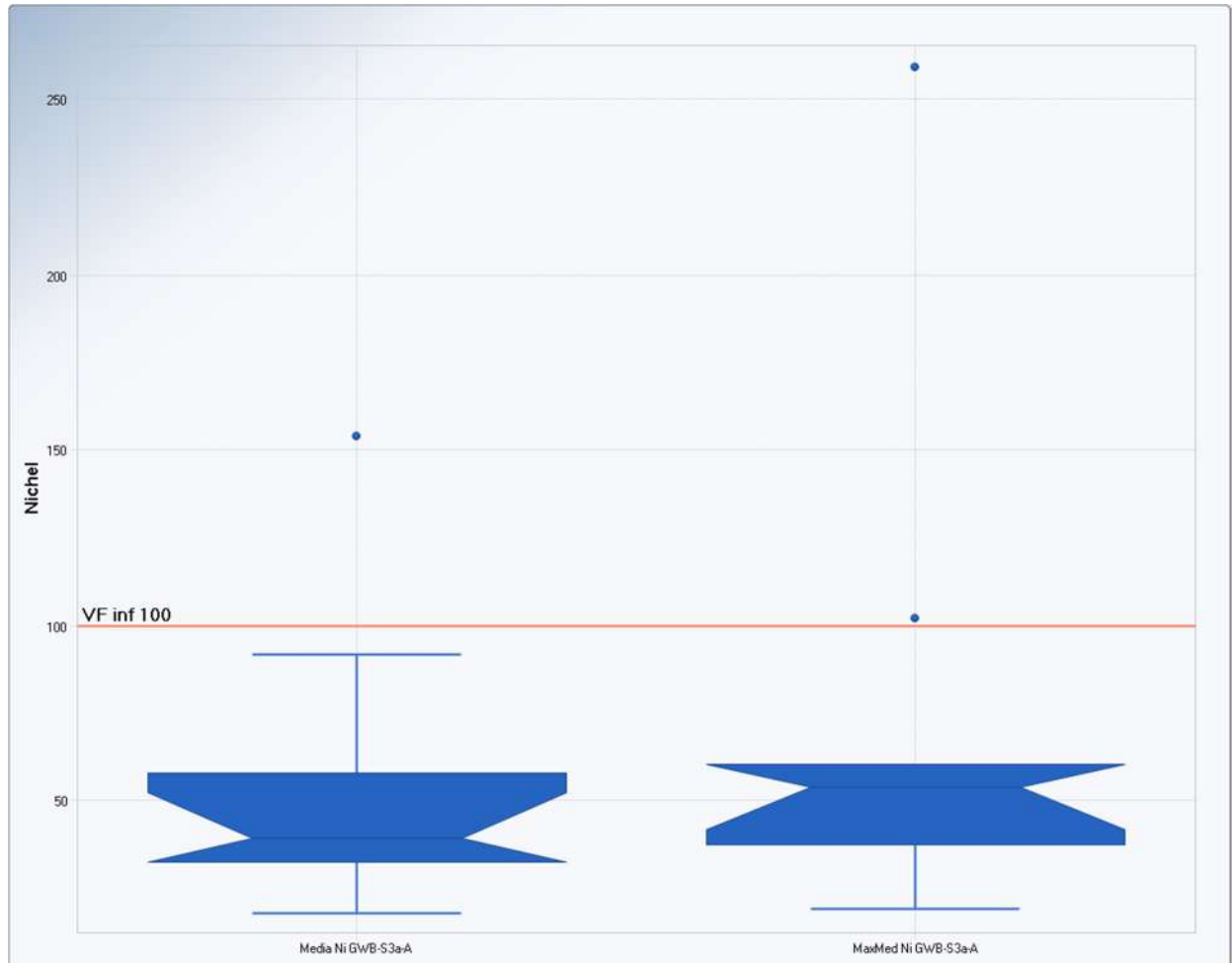
Figura 4.16: Box plot comparativo media e massimo della media per Nichel GWB-S3-A anni 2012-2016
