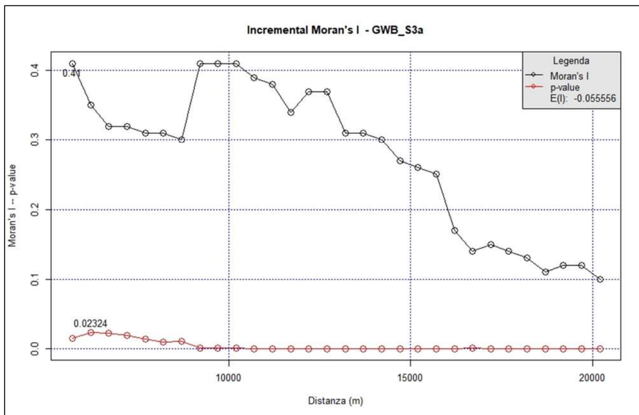
Figura 4.5: Analisi di autocorrelazione spaziale in GWB-S3a
