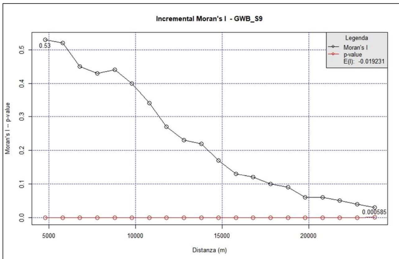
Figura 4.8: Analisi di autocorrelazione spaziale in GWB-S9
