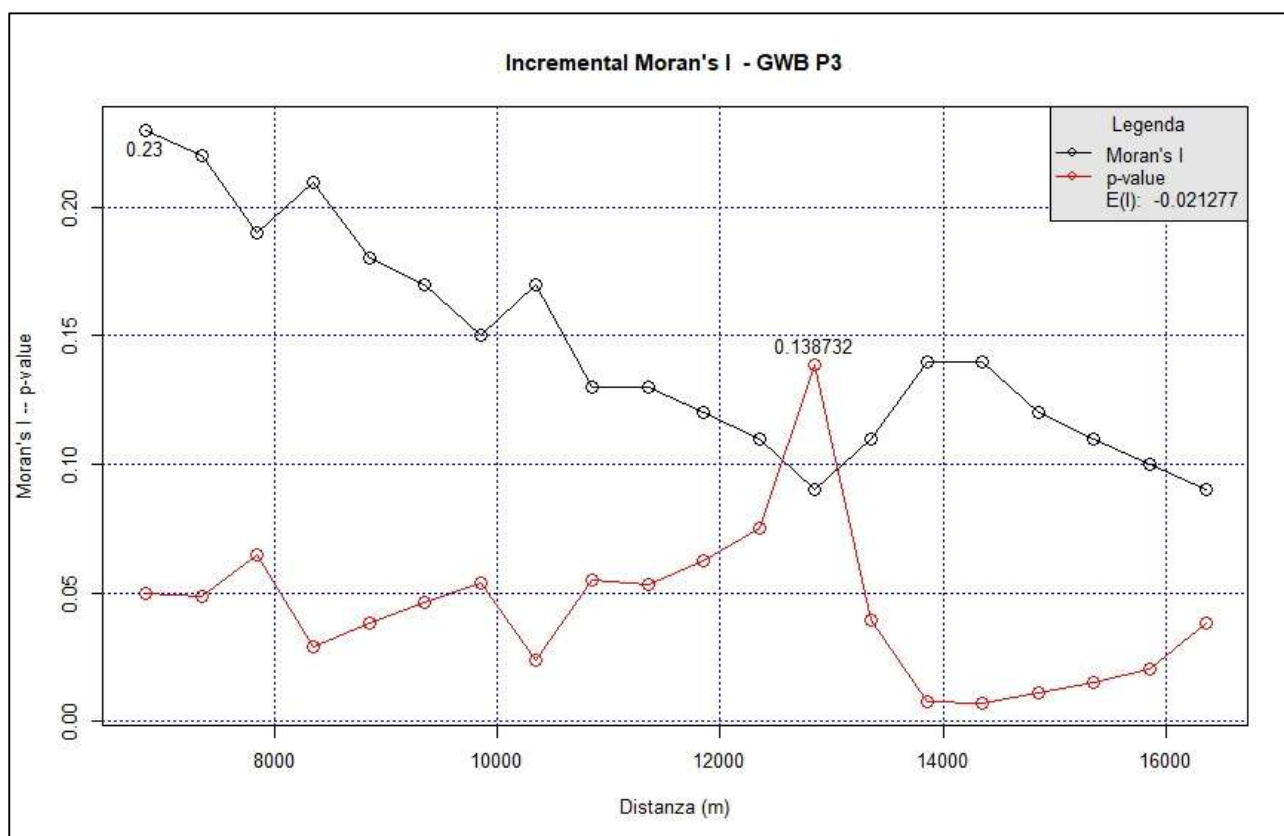
Figura 4.5: Analisi di autocorrelazione spaziale in GWB-P3
