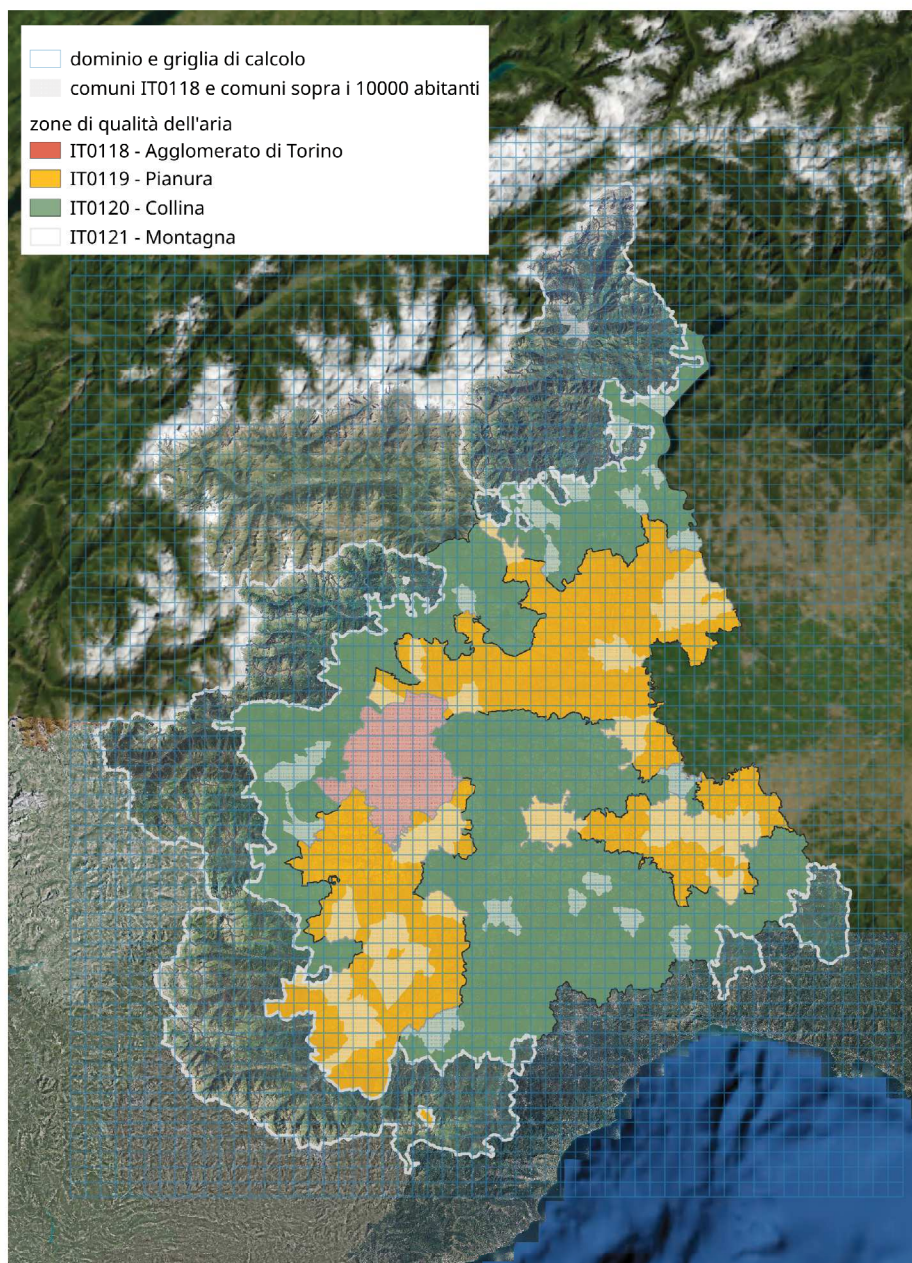
Figura 1. Zone di qualità interessate dai provvedimenti (IT0118, IT0119, IT0120), comuni interessati dai provvedimenti e griglia di simulazione del sistema modellistico
